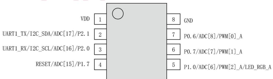
图 5-1-5 SOP8 封装引脚图
